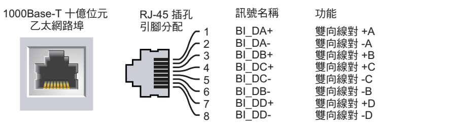
圖 6 十億元乙太網路埠引腳分配
