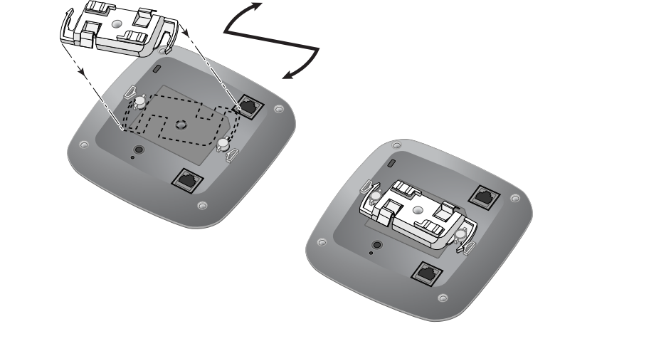
圖7 連接吊架軌道配接器
