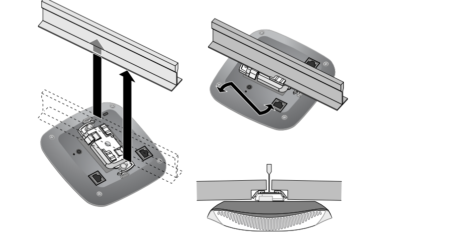
圖 8 安裝 AP
