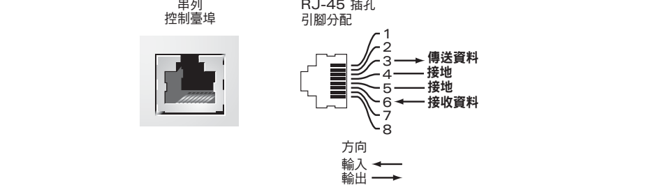
圖 5 串列埠引腳分配
